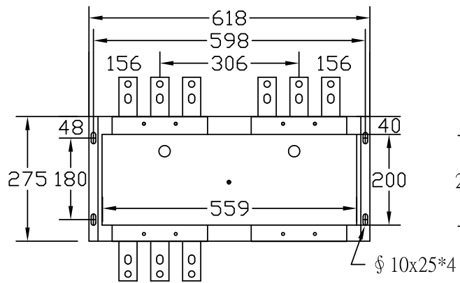
3P, 630AF/800AF
