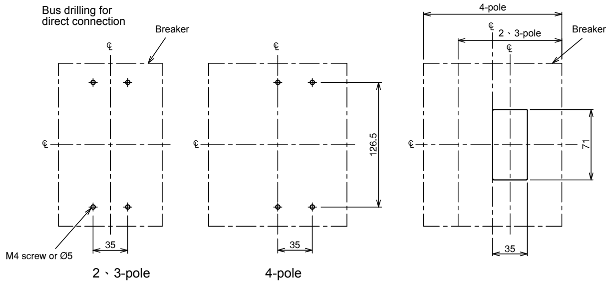
Front-panel cutout
