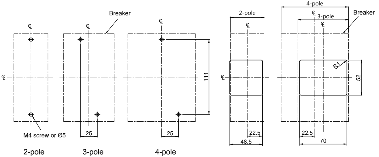
Front-panel cutout
